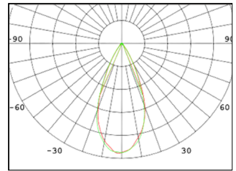
Symmetrical 45° F14504
