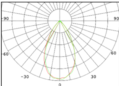
Symmetrical 60° F14505
